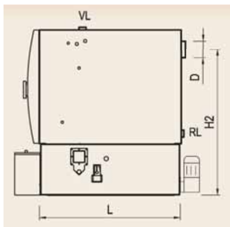
Descarga automática de cenizas con sinfín diagonal hasta el depósito de cenizas de 240 l
