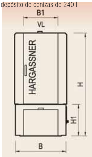
Descarga automática de cenizas con sinfín diagonal hasta el depósito de cenizas de 240 l
